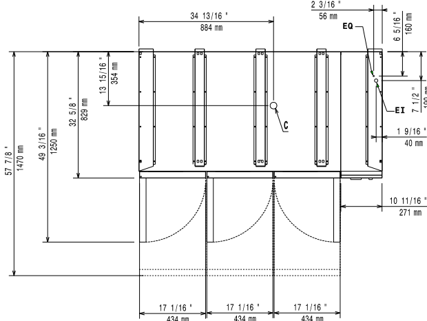
Boven aanzicht
